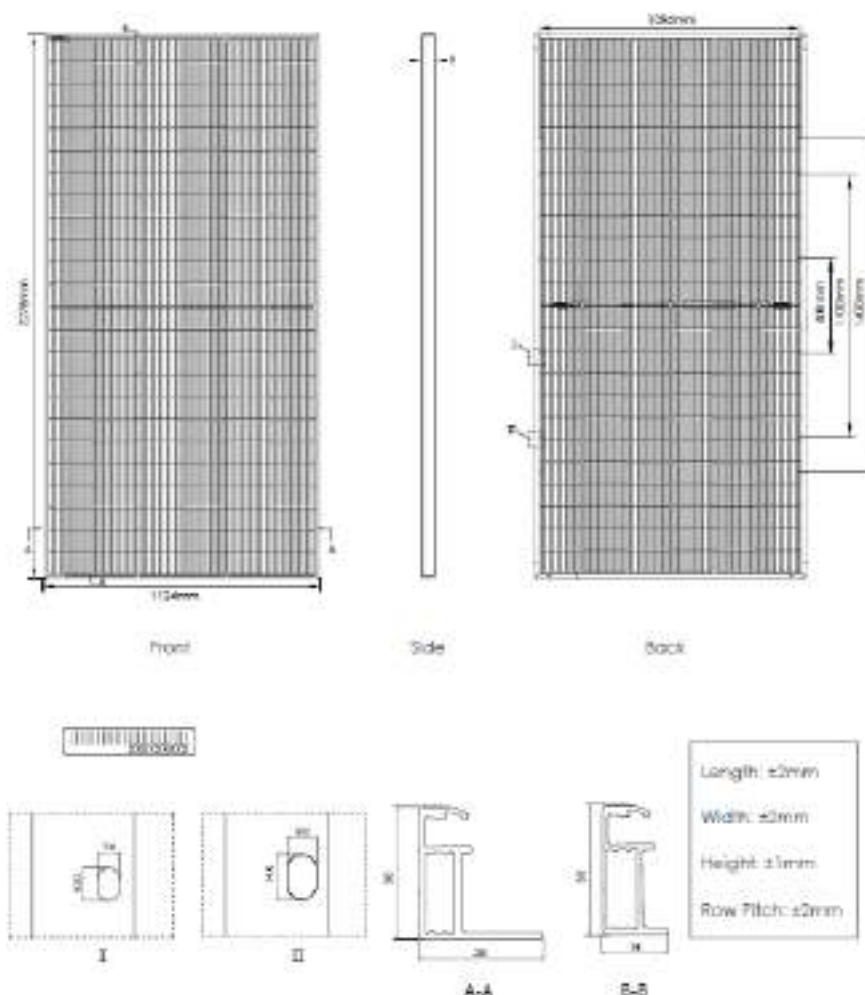
Imagen 2: Módulo Fotovoltaico Bifacial JKM570N-72HL4-BDV
